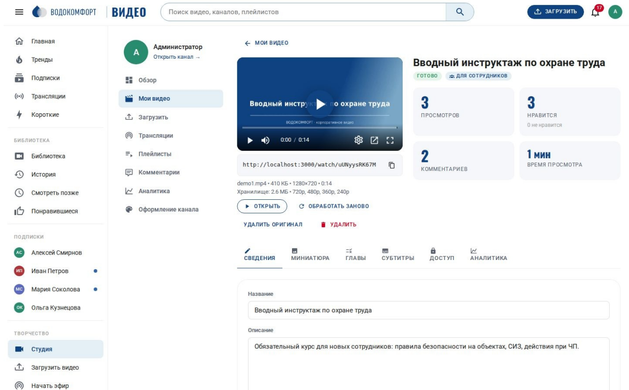
Рис. 34. Редактирование видео
