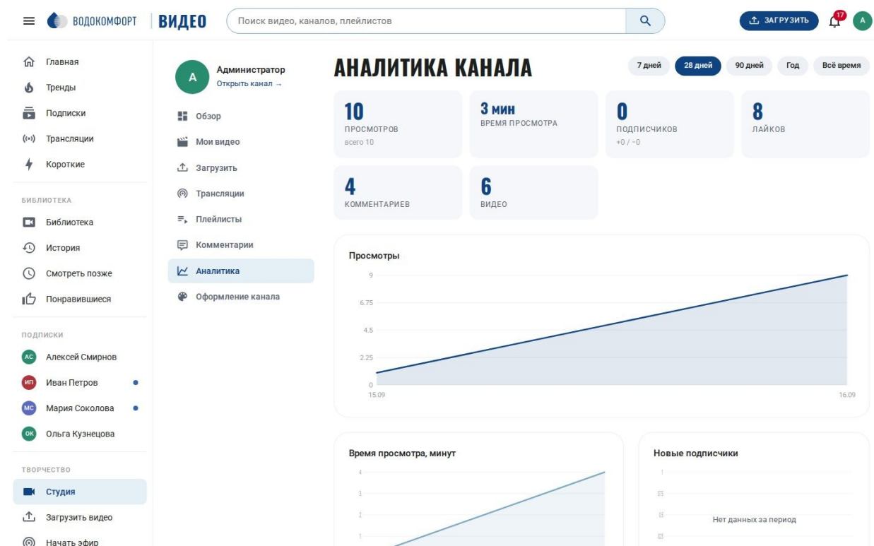
Рис. 35. Аналитика канала
